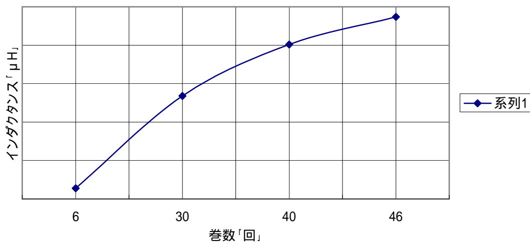
コイル巻数インダクタンスグラフ
